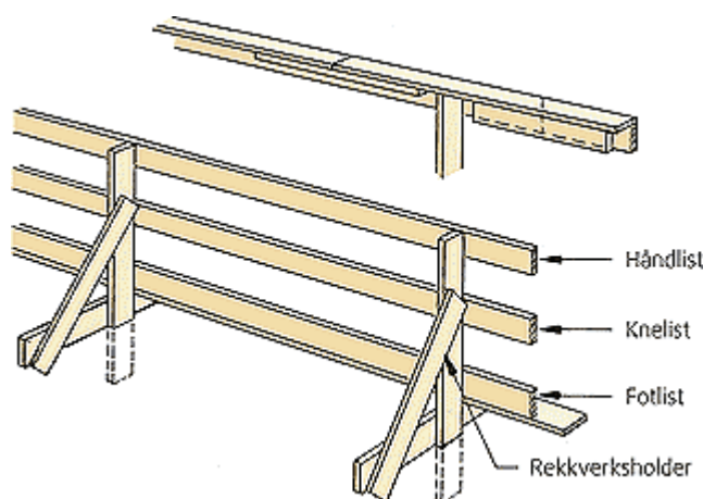
Fig. 222 Rekkverkets bestanddeler
