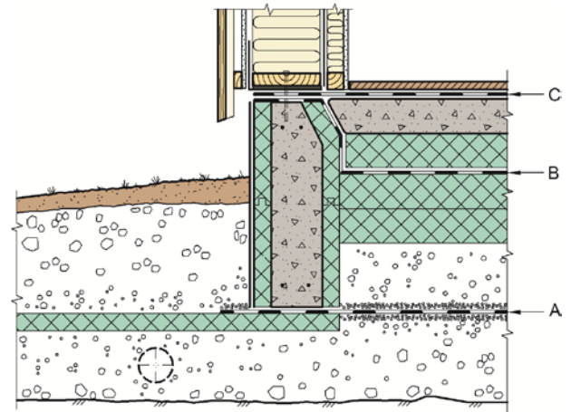
Fig. 1 Prinsipiell plassering av radonsperrer i ulike bruksgrupper. OLDROYD® Radontett RMA er godkjent i bruksgruppe A og B.
