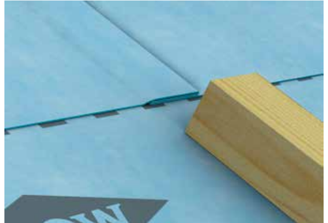
Fig. 7 Innbretting av duk ved skjøt
