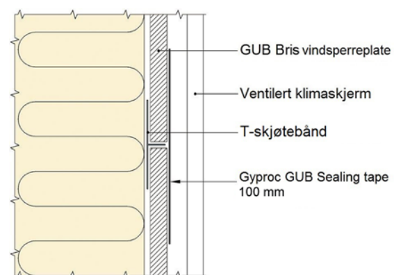
Fig. 5 Horisontal skjøt uten understøttelse med 100 mm Gyproc GUB Sealing tape montert sentrisk over skjøten.
