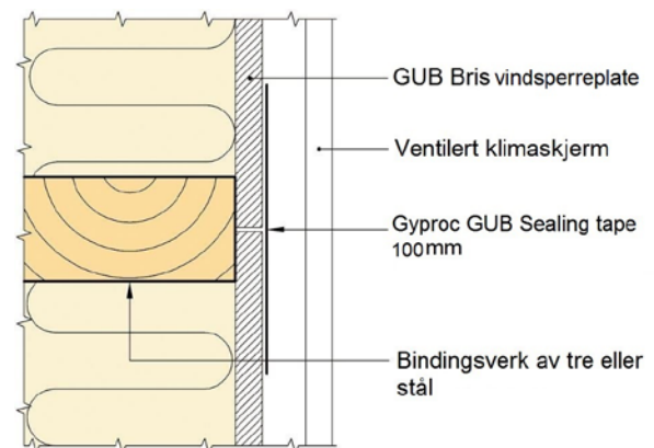
Fig. 4 Horisontal skjøt med understøttelse med 100 mm Gyproc GUB Sealing tape montert sentrisk over skjøten.
