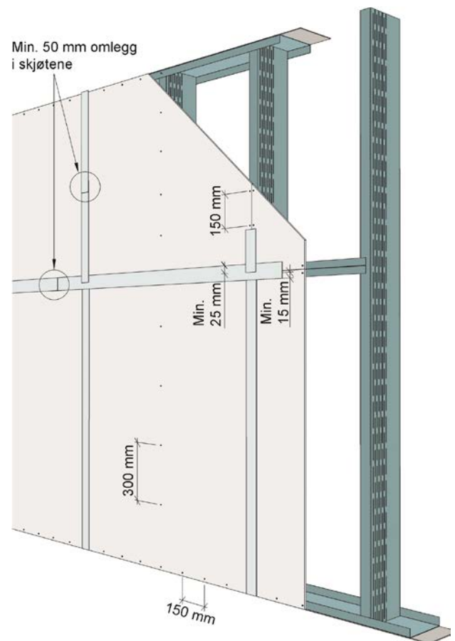
Fig. 1 Gyproc GUB Bris monteret på stendere av tynnplateprofiler i stål og med horisontalt T-skjøtebånd.
