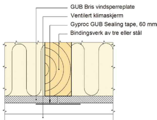
Fig. 2 Vertikal skjøt med Gyproc GUB Sealing tape 60 mm montert sentrisk over skjøten.
