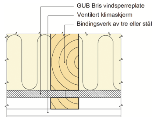
Fig. 3 Vertikal skjøt med klemler for Gyproc GUB Bris. Klemler festes med skruer c/c 250 mm.
